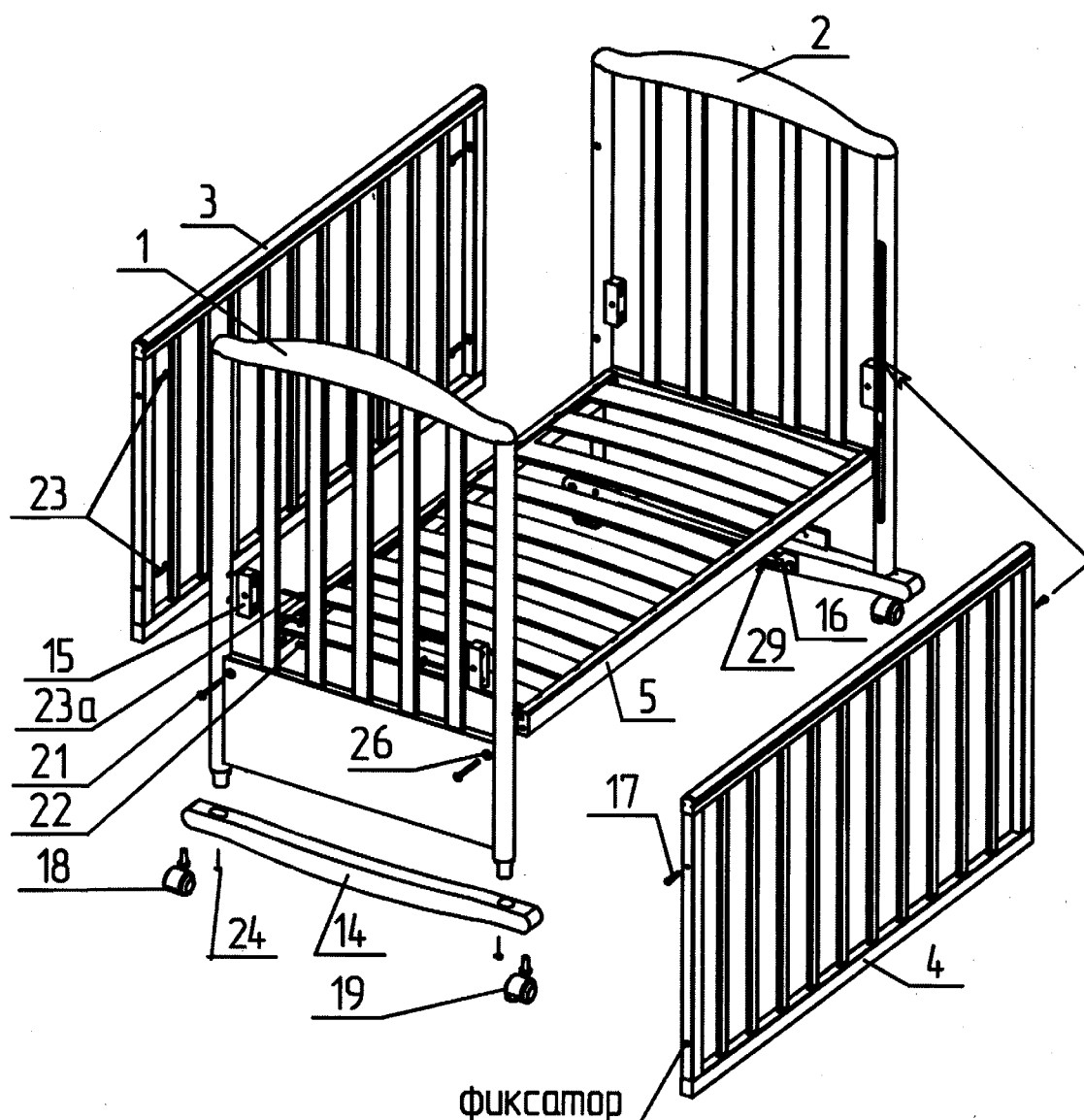
Схема сборки кровати. Рис.1
