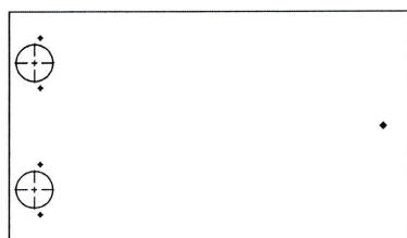
Я1 Панель передняя 890x190x16 (2 шт.)
