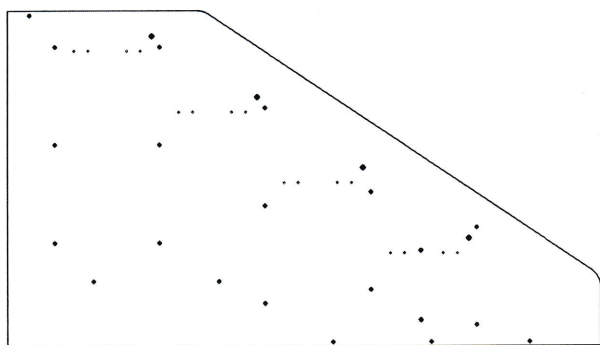
A17 Стенка задняя (774x386x16)-1 шт.
