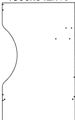
A4 Боковина левая 1360x842x16
