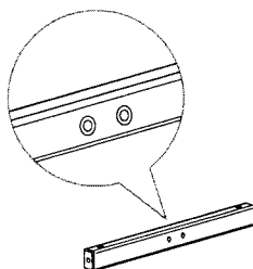
Распорка люльки под механизм привода L=380 мм (1шт.) O9
