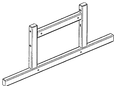
Рамка основания (2шт.) O1
