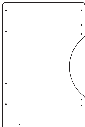
Боковина левая 1357x900x16
