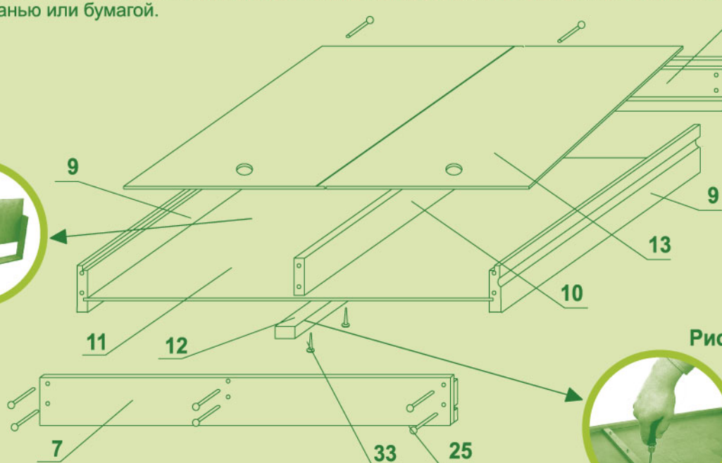
Схема 1: Сборка ящика.
